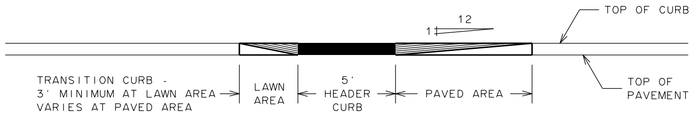
VIEW A-A
