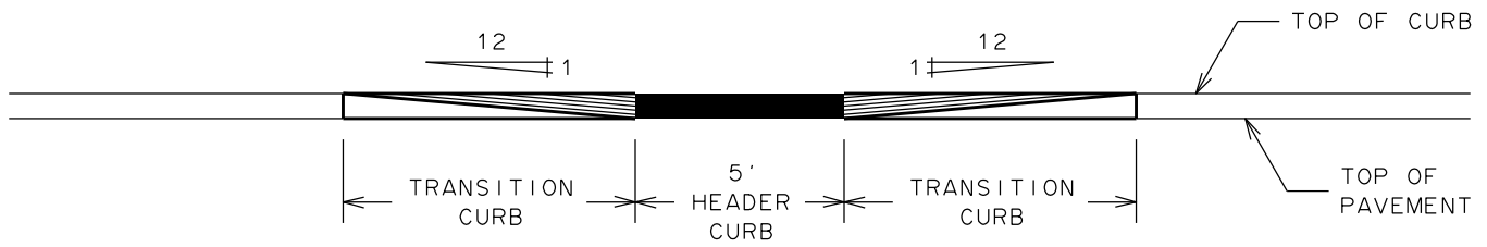
VIEW A-A
