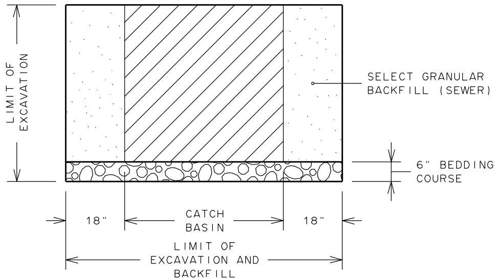
ELEVATION
