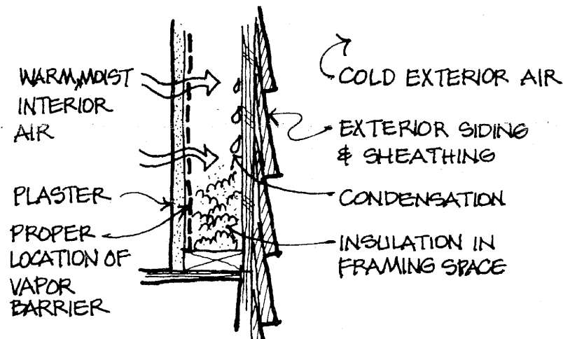
VAPOR BARRIER
